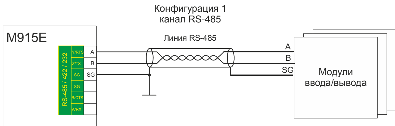
Рисунок 4 - Подключение внешних цепей к интерфейсу RS-485
