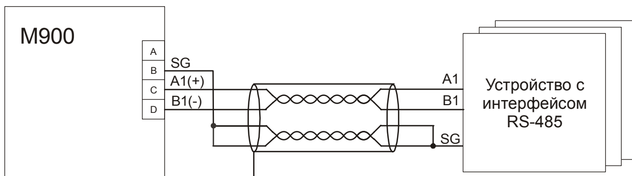
Рисунок 21 - Схема подключения с использованием кабеля с двойной витой парой
