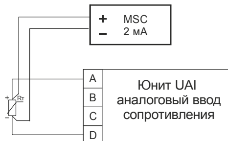
Рисунок 11 - Подключение термопреобразователя сопротивления по четырехпроводной схеме с внешним датчиком (MOPC-2MA) к юниту UAI
