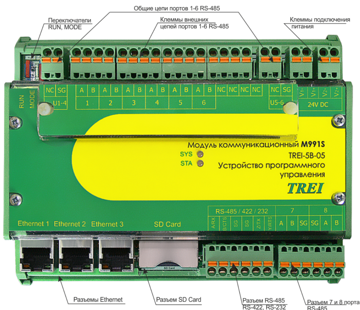
Рисунок 2 - Разъёмы и лицевая панель модуля M991S
