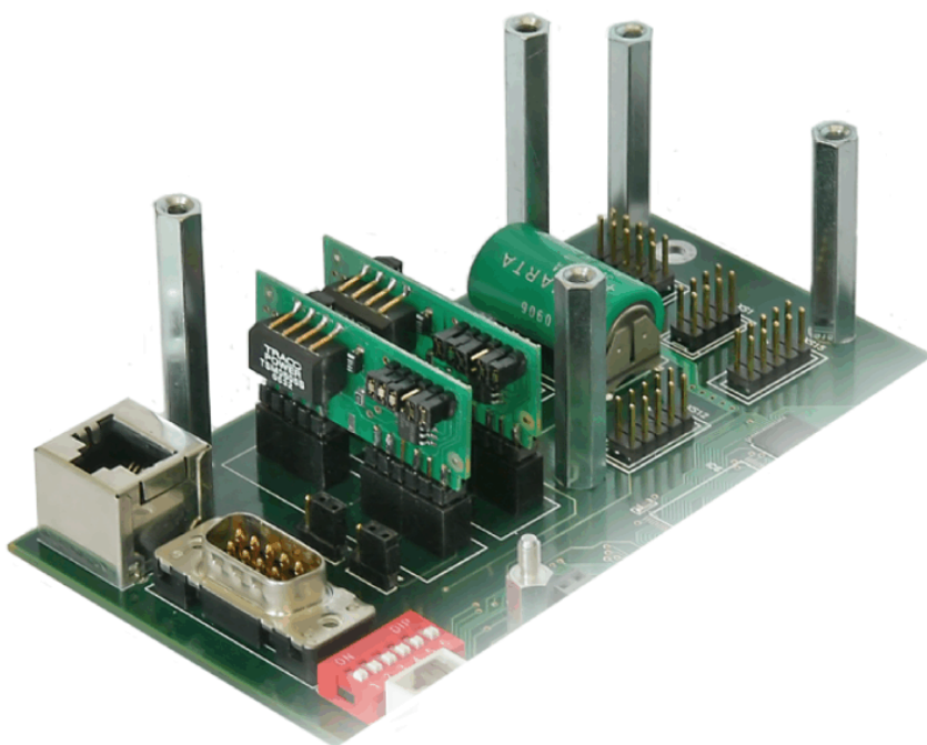
Рисунок 2 - Съемные юниты на плате мастера M902E
